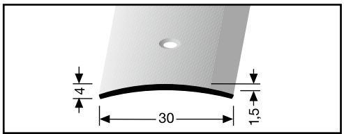
Übergangsprofil Easy 30 mm
