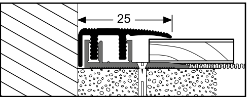
Click Endprofil 6 - 10 / 15 / 20 mm
