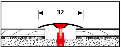
Fix Übergangsprofil 0-20 mm
