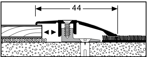
Schraub Ausgleichsprofil 6,5 - 16 / 26 mm
