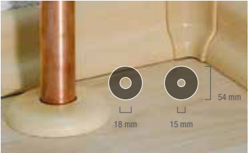
Heizrohrrosetten
