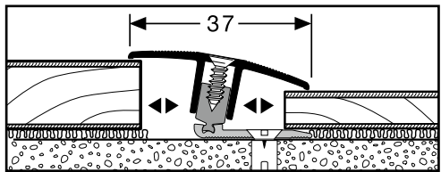
Schraub Übergangsprofil 7-17 / 27 mm
