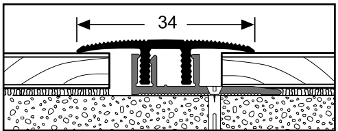
Click Übergangsprofil 6 - 10 / 15 / 20 mm
